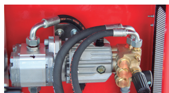
Nettoyeur haute pression intégré.
